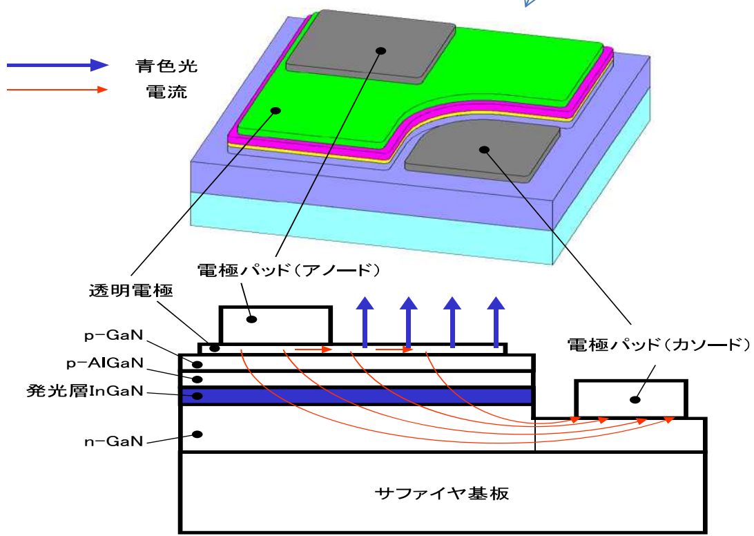
図 3. LEDチップ
