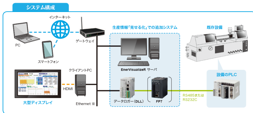
エネルギーと生産情報「見える化」のシステム構成
