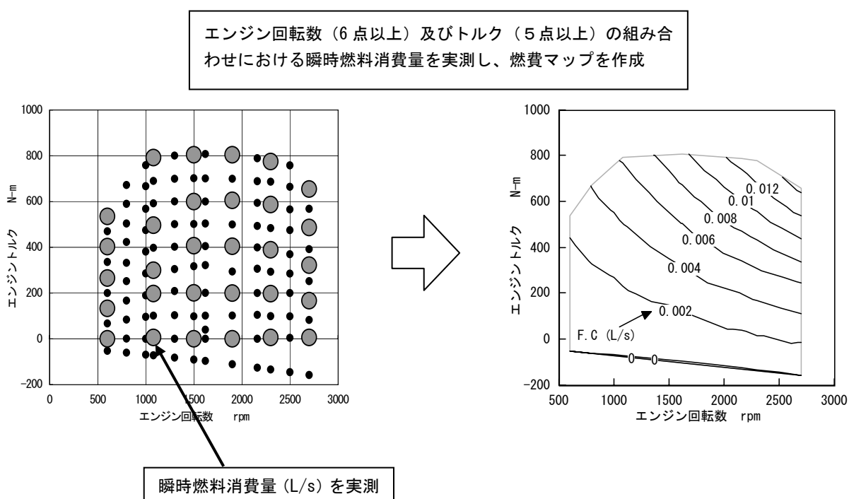
図 エンジン燃費マップの作成手順
