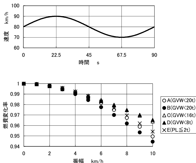
図1 速度変動が燃費に及ぼす影響
