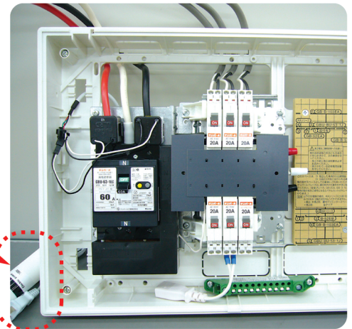
▲ 分電盤にセンサを設置(例)
